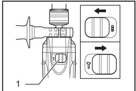
► 1. Action mode change lever
