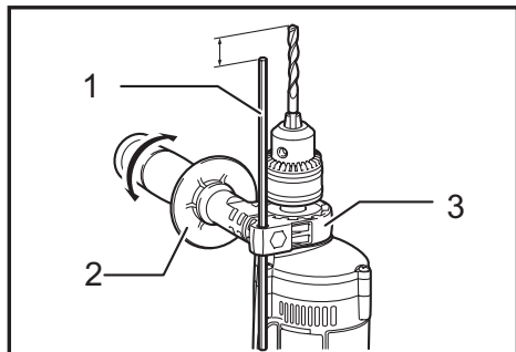
► 1. Calibrador de profundidad 2. Empuñadura lateral 3. Base de la empuñadura
